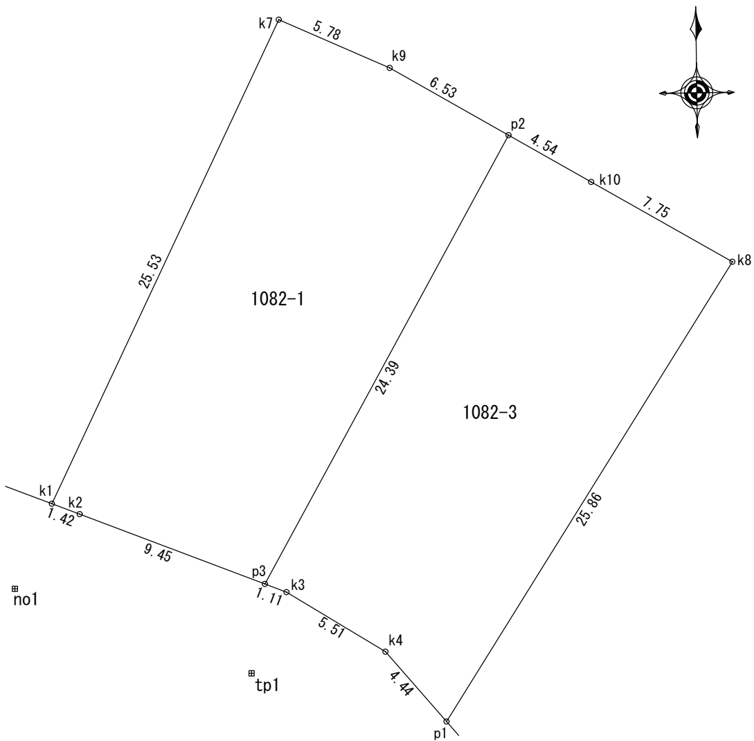
求積表
